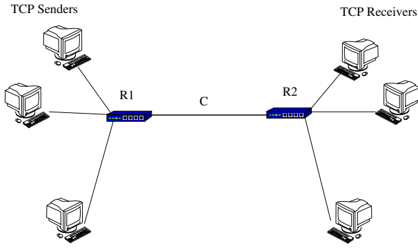
Fig. 2. Simulation scenario.
